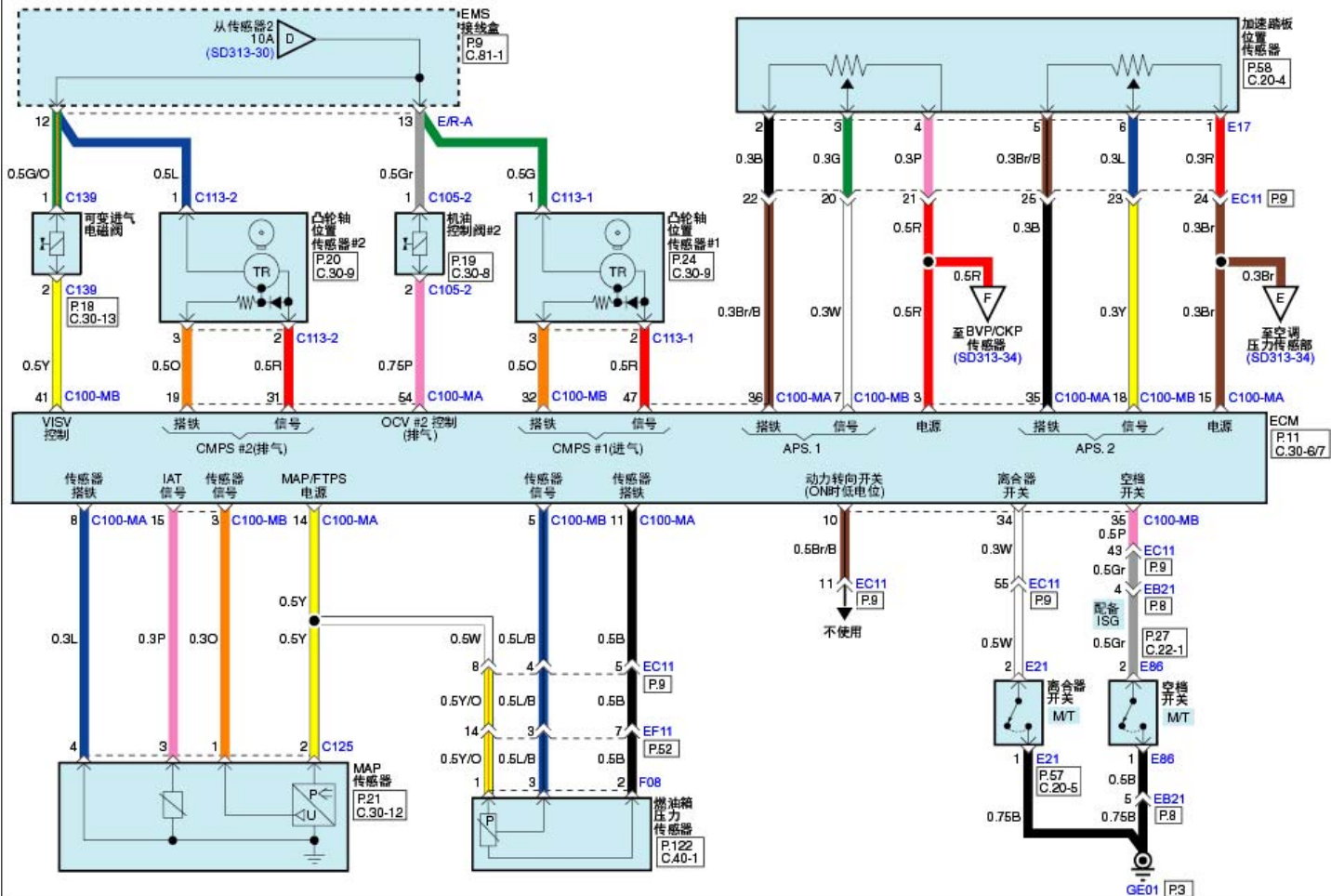
发动机控制系统(G4FG : GAMMA 1.6L MPI M/T - 配备欧6)(6)
